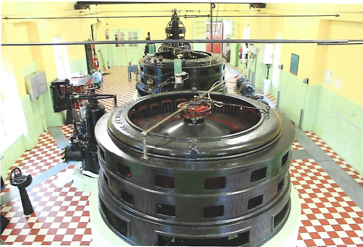
Stil på industribyggnaderna förr i världen. Sälbodas turbinhall. Se artikel s 6-7. Foto: Tess
